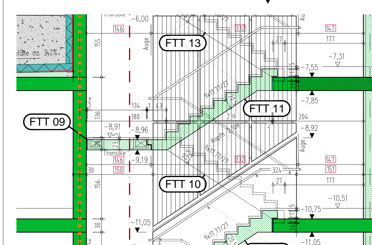
TREPPE FTT 09 | 10 | 11 SCHNITT S2 - 1:50
